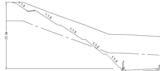
<A-A'단면>
