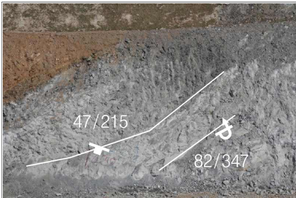
【그림 23】 C 영역 상세사진 (불연속면 발달)
